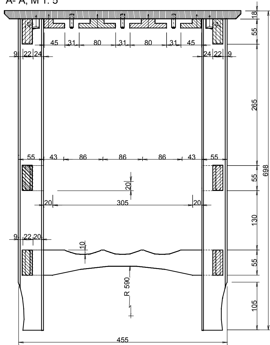
A-A, M 1: 5
