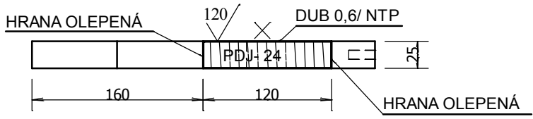
A - A, M 1: 5
