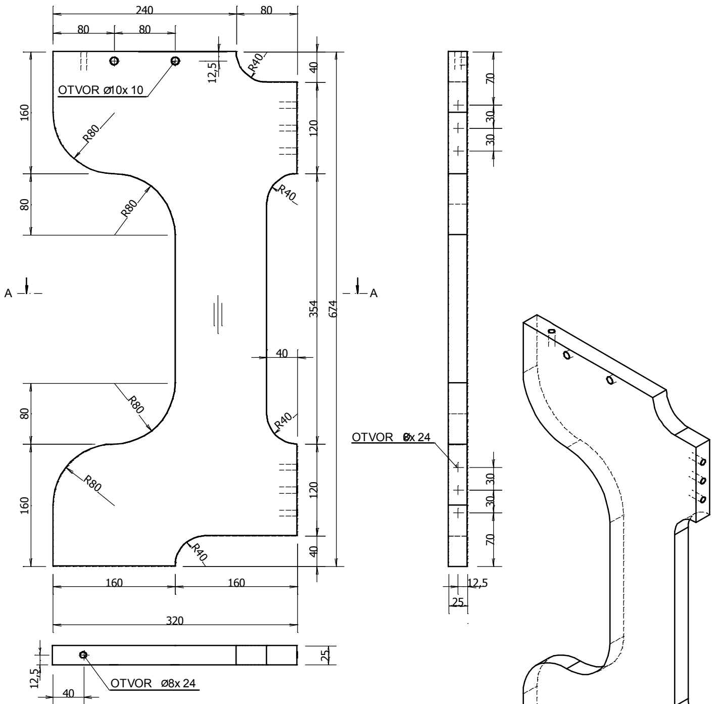
A - A, M 1: 5
