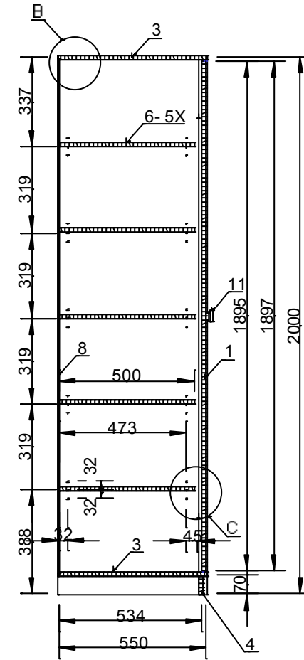
A-A, M 1:20
