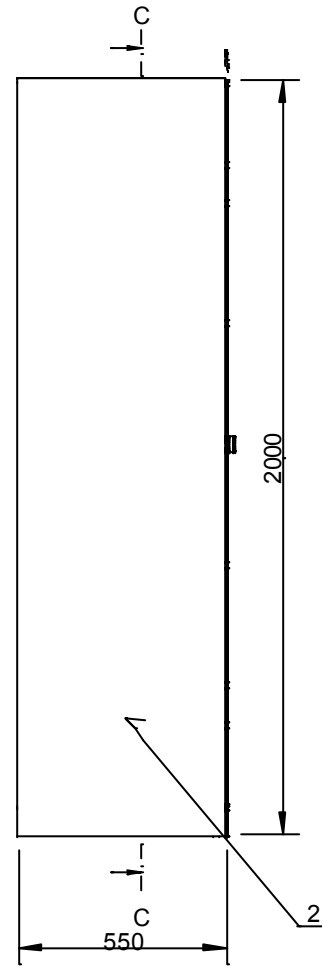
POHLAD-BOČNÝ, M 1:20
