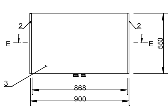
POHLAD-PÔDORYSNÝ, M 1:20
