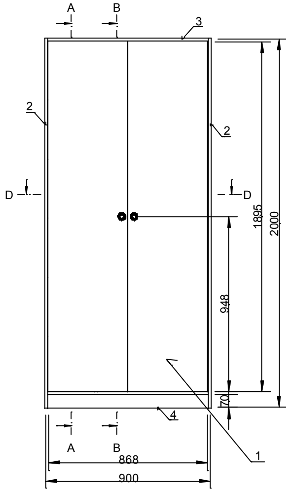
POHLAD-ČELNÝ, M 1:20
