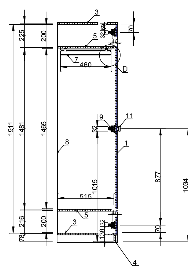
B-B, M 1:20
