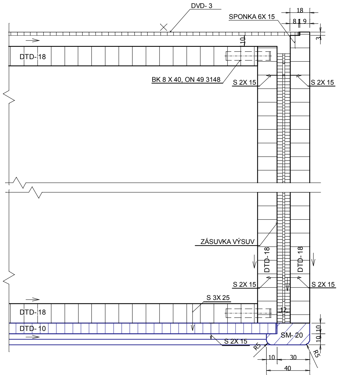
A-A, M 1:2
