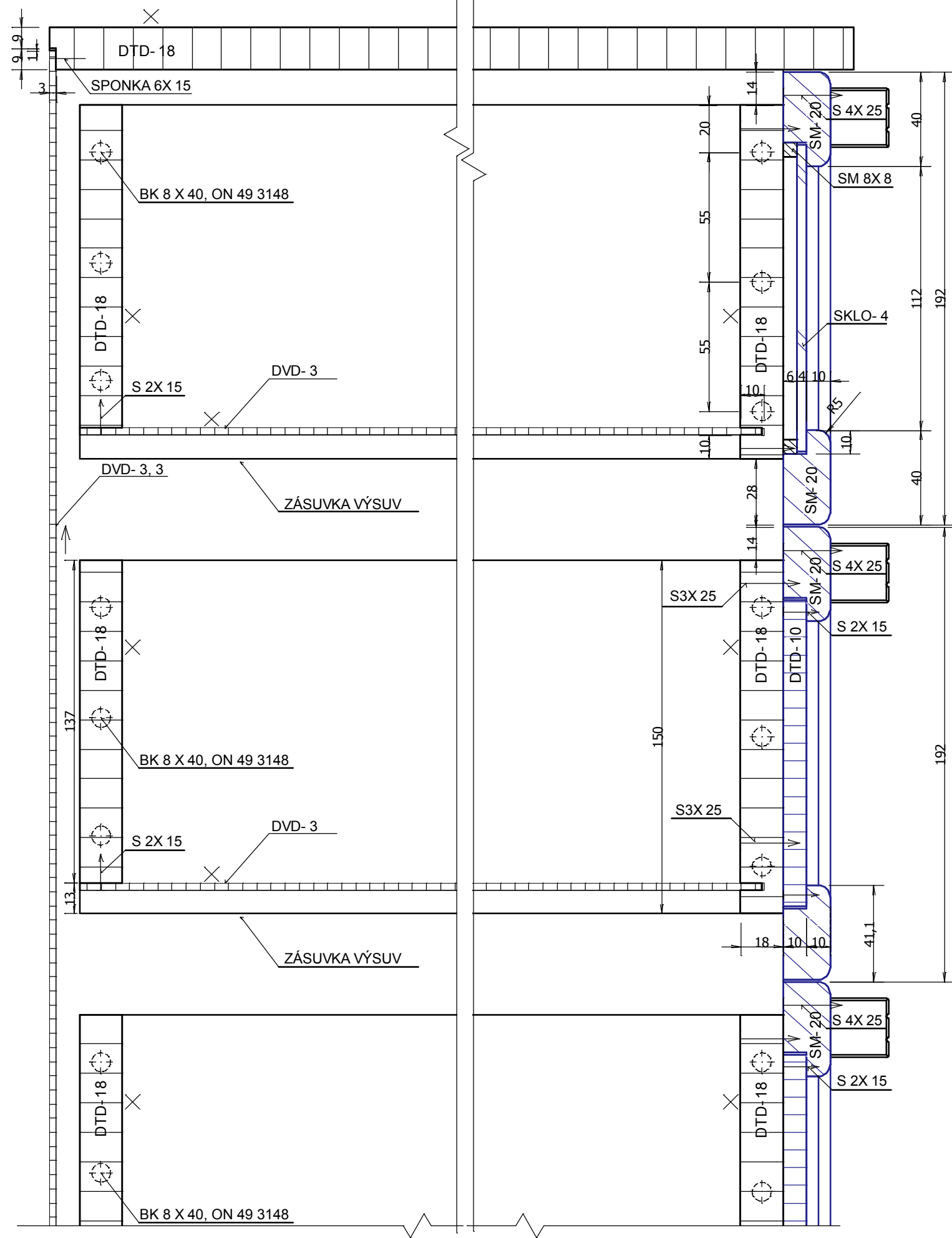
B-B, M 1:2
